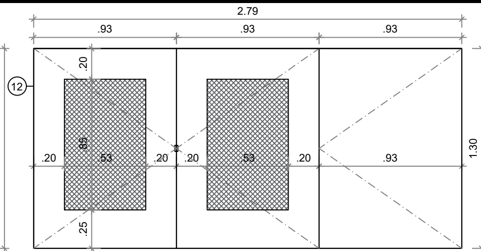
ESQUEMA DE PORTA TRIPLA COM ABERTURA TELADA PARA VISUALIZAÇÃO DE HIDRÔMETRO
